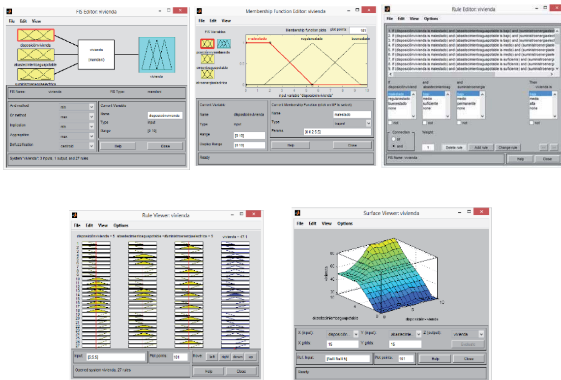
Figura 4. Editores y visores de Matlab. Fuente: Matlab
