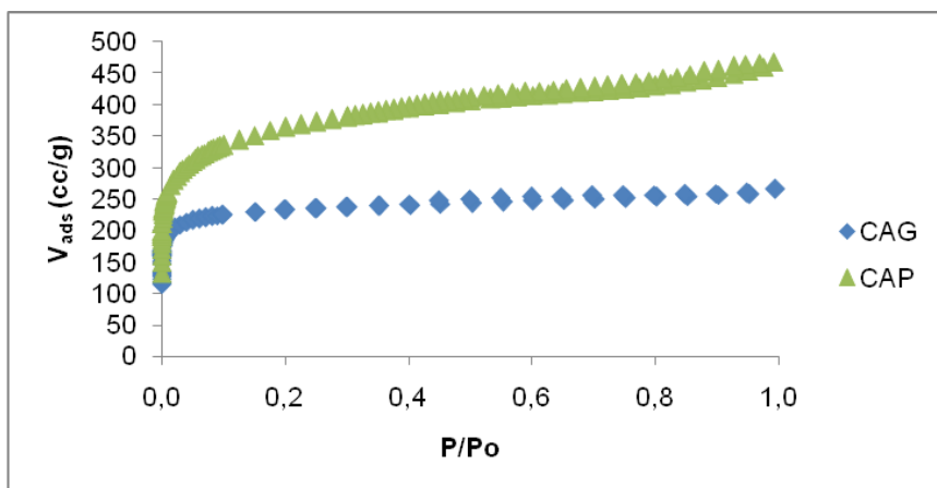
Figura 4. Isoterma de adsorción-desorción de nitrógeno a 77K para las dos muestras carbonosas (CAG y CAP).
