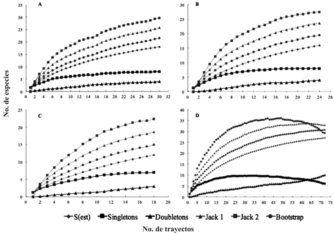
Figura 2. Curva de acumulación de especies del área de bosque (A), sistema silvopastoril (B), área de minería (C) y (D) acumulado en el paisaje, usando los estimadores Jackknife 1, Jackknife 2, Bootstrap, Singletons y Doubletons.
